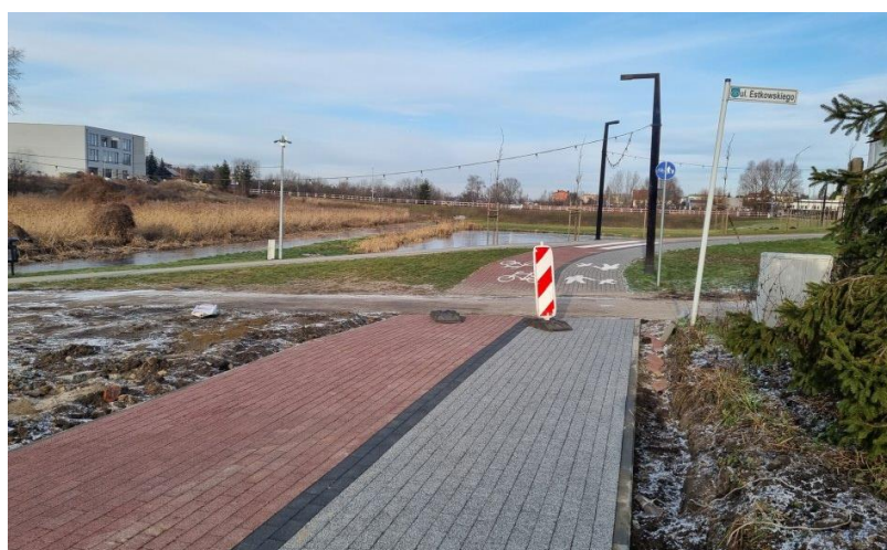
Ścieżka pieszo-rowerowa łącząca ulicę Estkowskiego z ulicą Średzką w Kostrzynie
